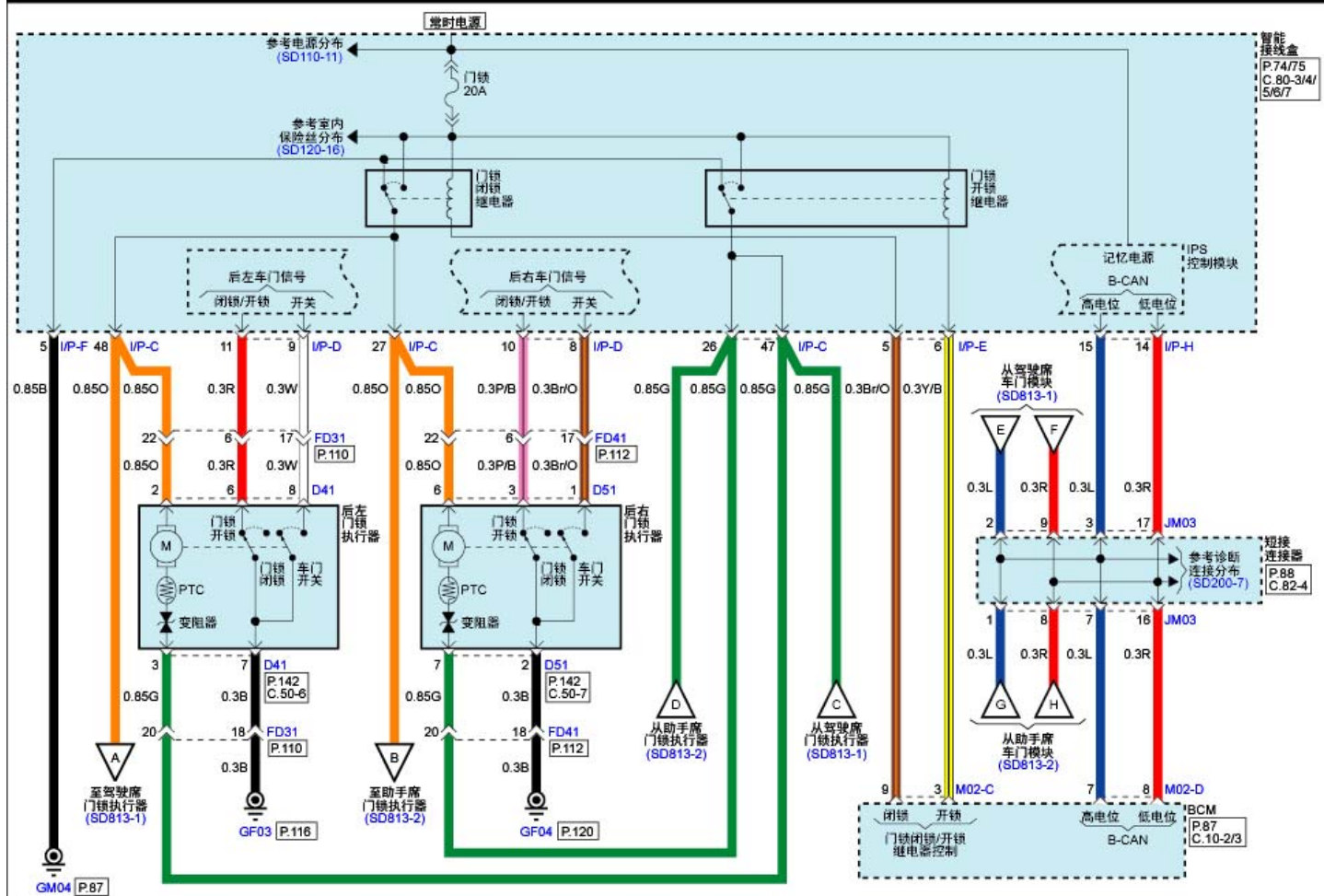
电动门锁(3)
